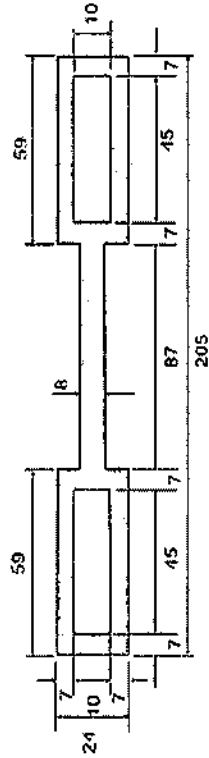
Diseño y dimensiones de la contra asa:
