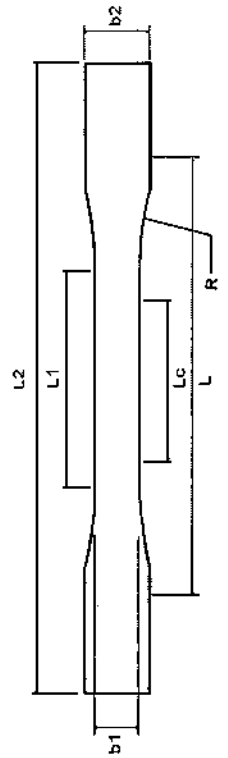
Espécimen de ensayo: Tipo I moldeado con el compuesto plástico que se solicita en la producción de la asa y contra asa
